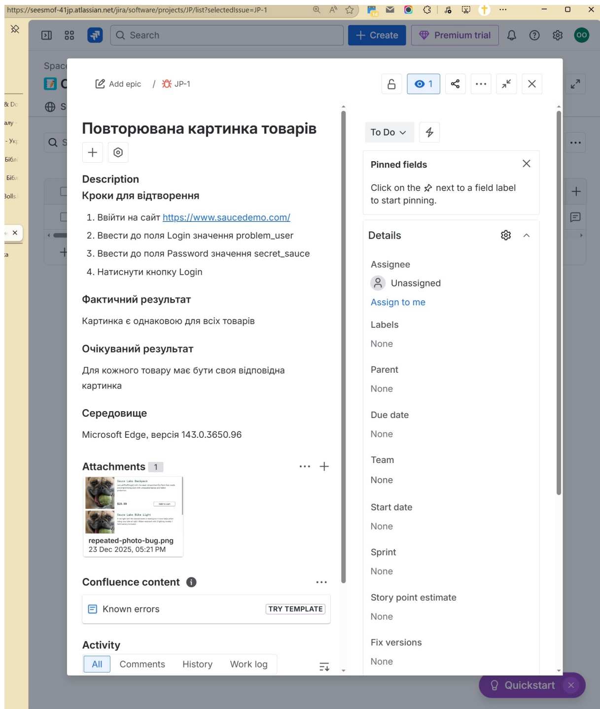
Рисунок 1.5 — Доданий баг-репорт
