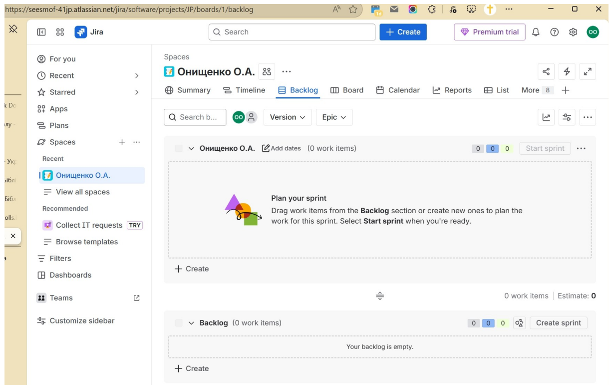
Рисунок 1.4 — Вигляд дошки
